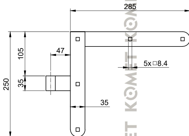
Zawias górny
