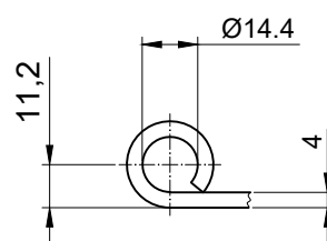
Szczegół A Skala 1:2
