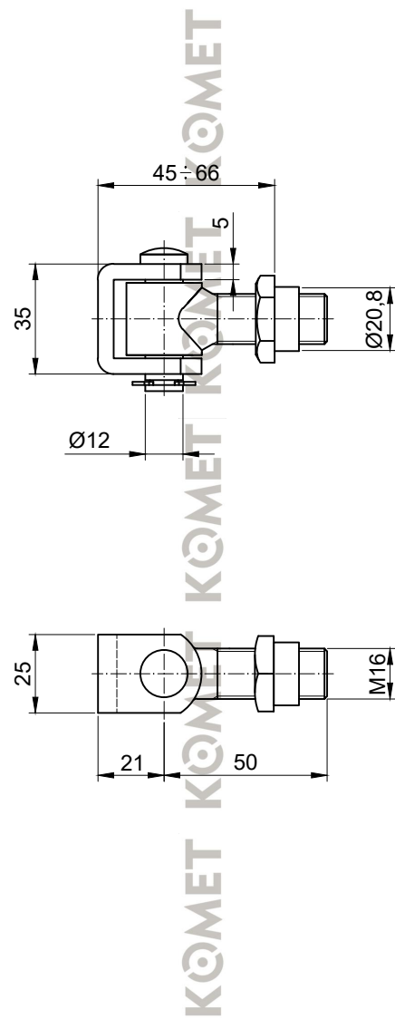
KOMET Zawias regulowany M16 z tulejką do przyspawania
