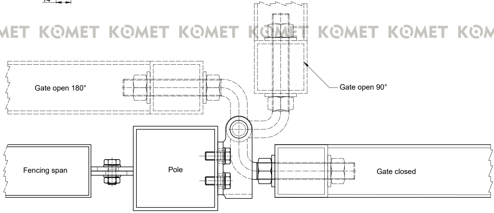
KOMET Adjustable hinge M16 L-125 bent 180° W71553
